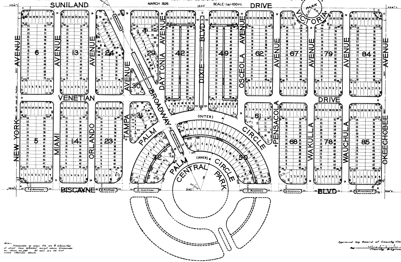
KEY MAP
